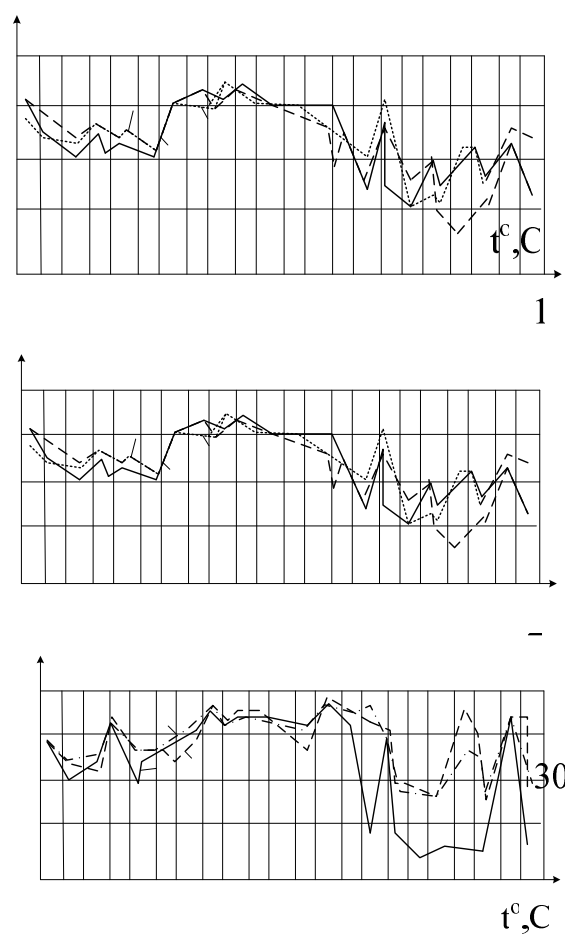
Fig. 5. Variația temperaturii aerului pe verticală la: a - sistemul de răcire cu aer; b - sistemul de răcire indirectă a aerului instalat în partea de sus a depozitului; c - sistemul de răcire indirectă a aerului instalat la pereții depozitului; 1 - la înălțimea 0,25 m; 2 - la înălțimea 2,0 m; 3 - la înălțimea 4,0 m.
