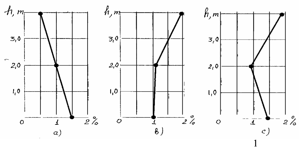
Fig. 6. Variația pierderilor de greutate a merelor "Calvil" în depozite cu: a - sistem de răcire indirectă a aerului instalat în partea de sus a depozitului b - sistem de răcire indirectă a aerului instalat la pereții depozitului c - sistem de răcire cu aer
